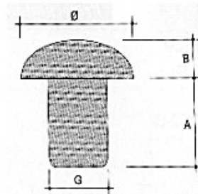
PARACOLPI TESTA BOMBATA \varnothing 24 mm in polietilene
