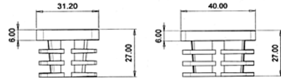
PUNTALE ALETTATO QUADRO 30x30 - 40x40 in polietilene
